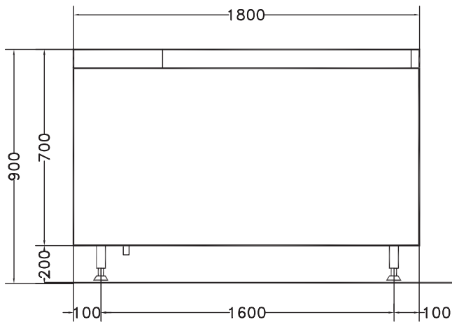
Zij aanzicht
